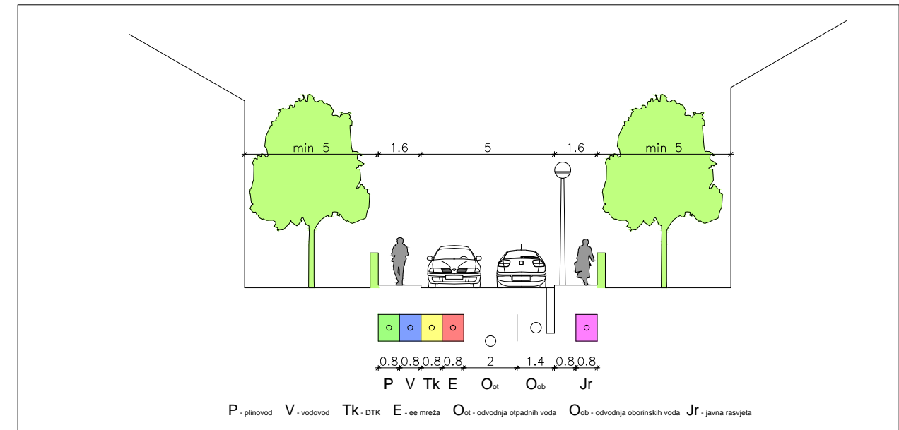
KARAKTERISTIČNI POPREČNI PROFIL PLANIRANE PROMETNICE m. 1:200
