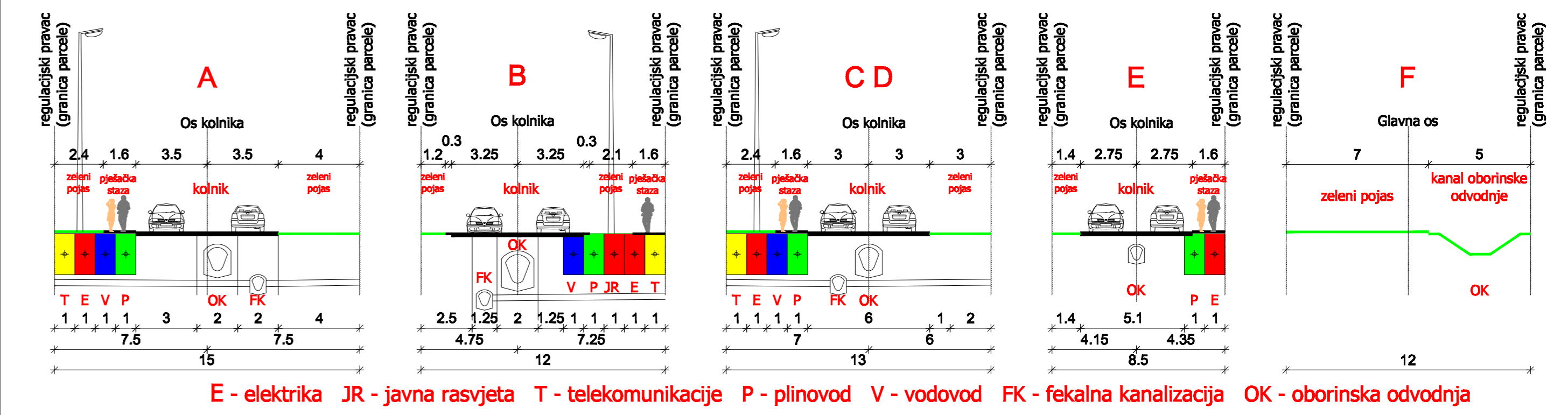
POPREČNI PROFIL PLANIRANIH ULICA - m.1:200
